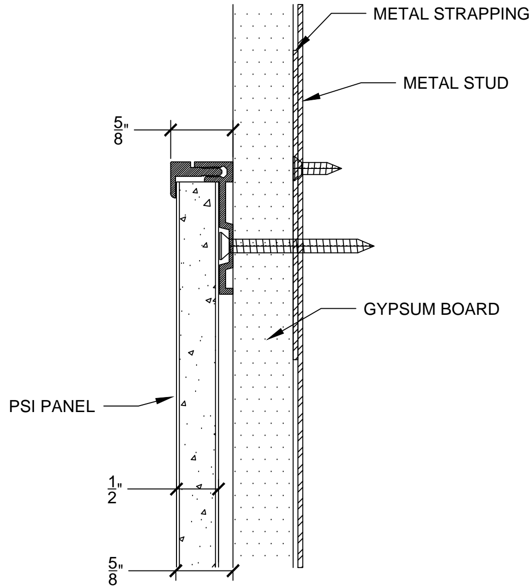
#610A TOP EDGE TRIM
