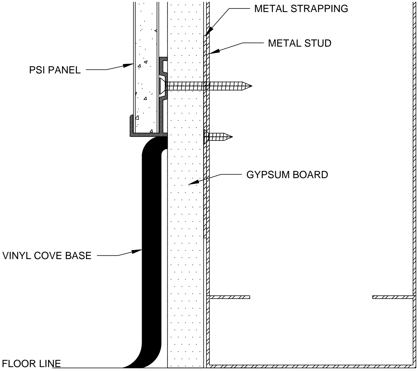
#610 BOTTOM EDGE TRIM - ABOVE BASE
